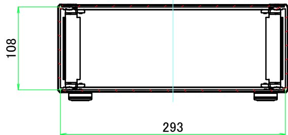
A-A (1:5)
